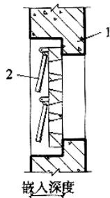
图 3.4.6 悬板活门嵌入墙内深度示意
