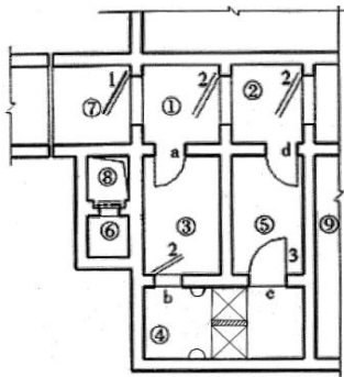
图 3.3.23 洗消间平面
